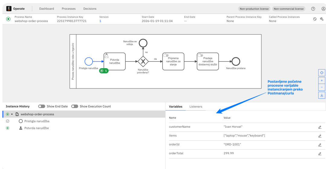
Slika 34. Procesna instanca “webshop-order-process” u Camunda Operate aplikaciji s početnim procesnim varijablama definiranim putem REST API-ja.
